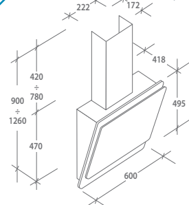
ESQUEMA ENCASTRE (mm)
