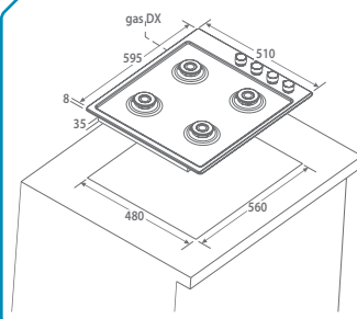
ESQUEMA ENCASTRE (mm)
