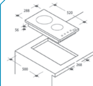
ESQUEMA ENCASTRE (mm)
