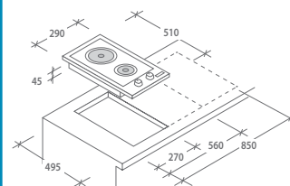
ESQUEMA ENCASTRE (mm)
