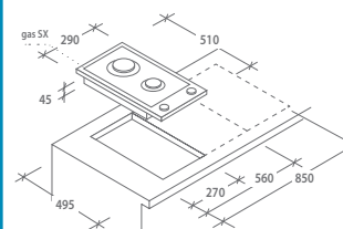
ESQUEMA ENCASTRE (mm)
