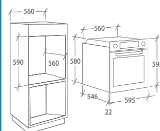
ESQUEMA ENCASTRE (mm)
