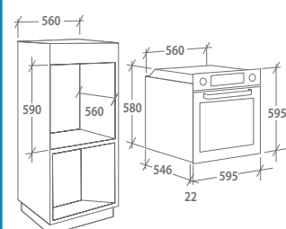
ESQUEMA ENCASTRE (mm)
