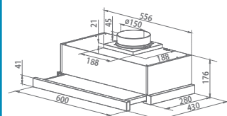
ESQUEMA ENCASTRE (mm)
